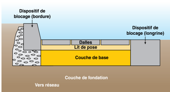
Exemple de dispositif de blocage de rive
