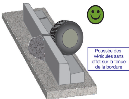
Exemple de calage par épaulement
